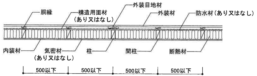
水平断面図
