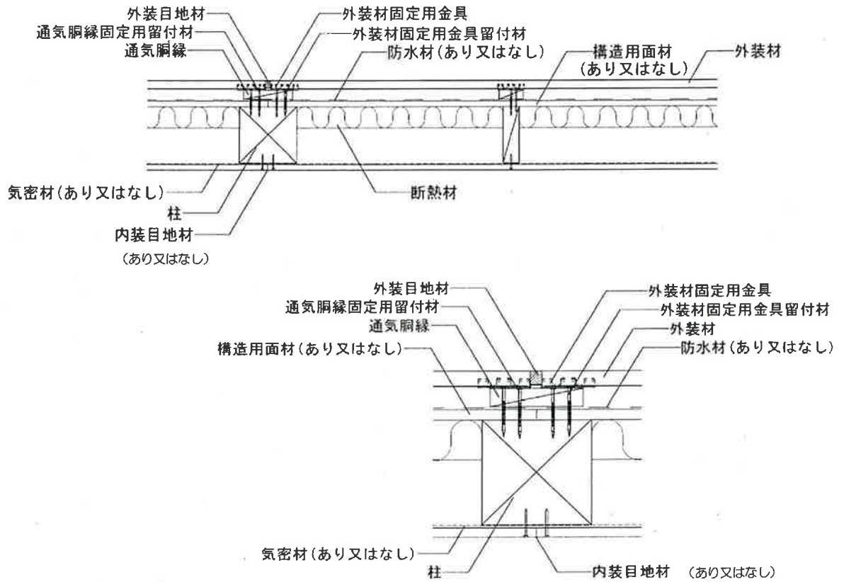
水平断面図
