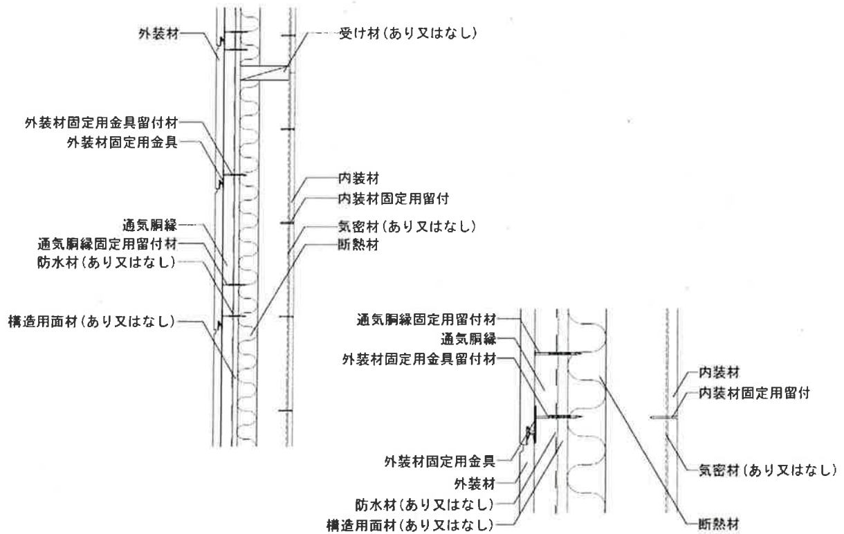
鉛直断面図
