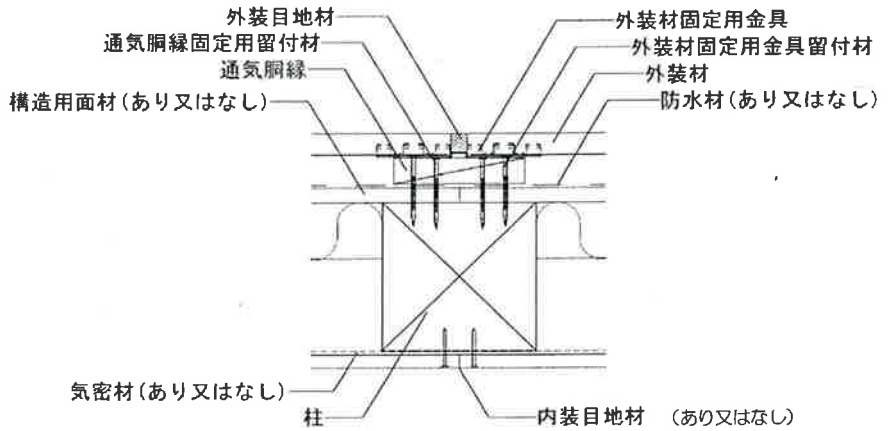
水平断面図
