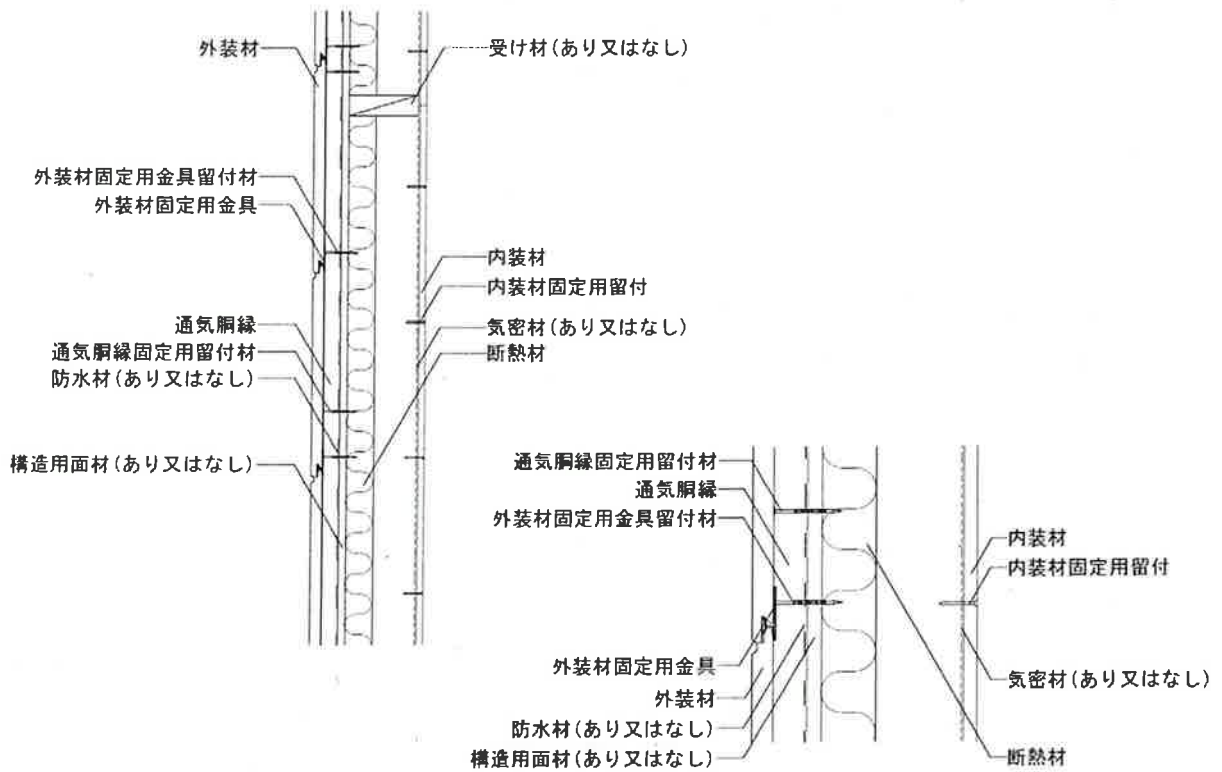
鉛直断面図
