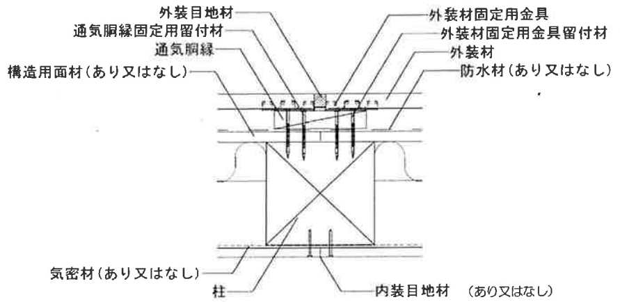
水平断面図
