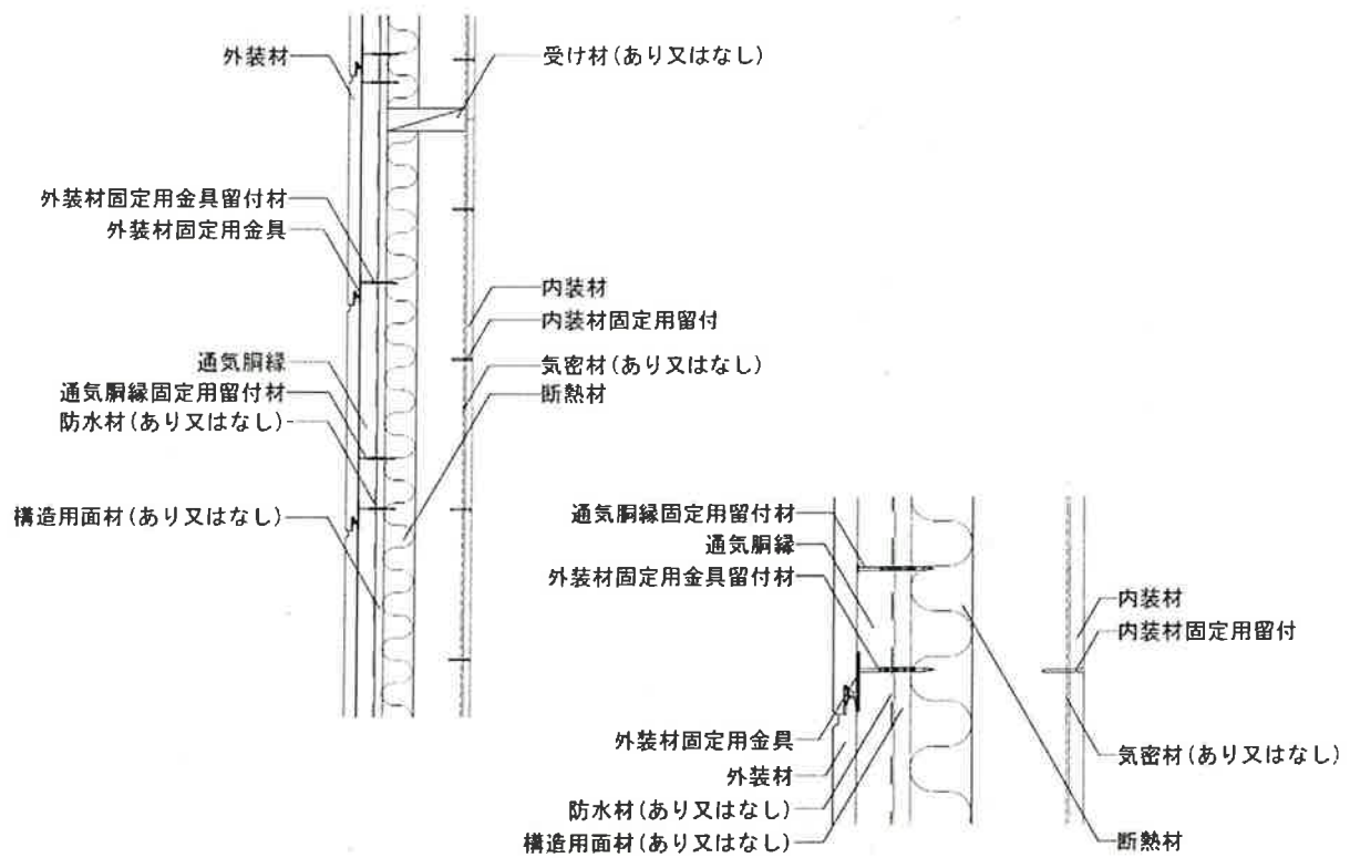
鉛直断面図
